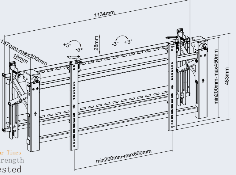
帶彈出式系統安裝 VESA JW03-48T 54"-70" 70kg/154lbs 137-300mm 200x200 400x200 300x300 400x400 600x400 800x400
